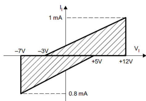
شکل ۱. مدار آزمون اندازه گیری UL برای RS485 شکل ۲. رابطه و حدود جریان و ولتاژ برای UL=1
