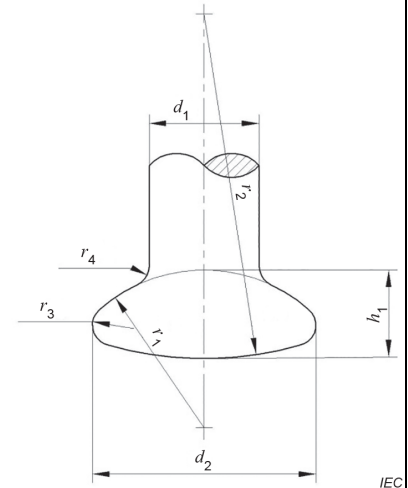
شکل ((۷-۱)): یراق بال
