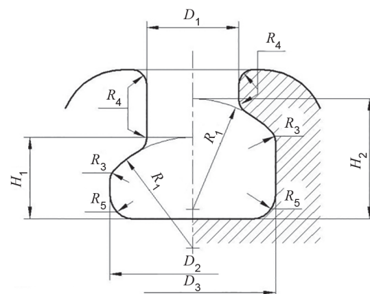
شکل ((۷-۲)): یراق سوکت
