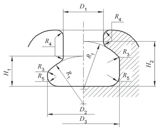
شکل ((۷-۲)): یراق سوکت
