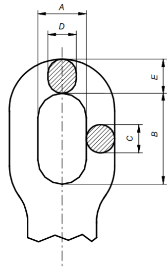
شکل ((۷-۳)): یراق آی
