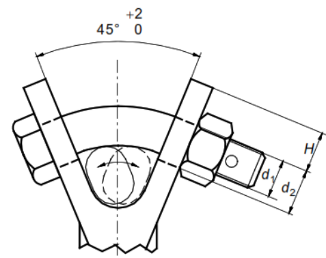
شکل ((۷-۳)): یراق وای کلویس
