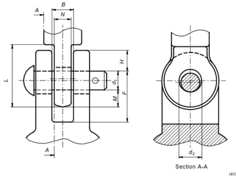
شکل ((۷-۲)): کوپلینگ تانگ و کلویس
