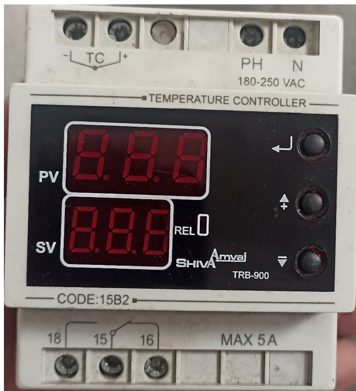
شکل ۱: کنترلر دما
