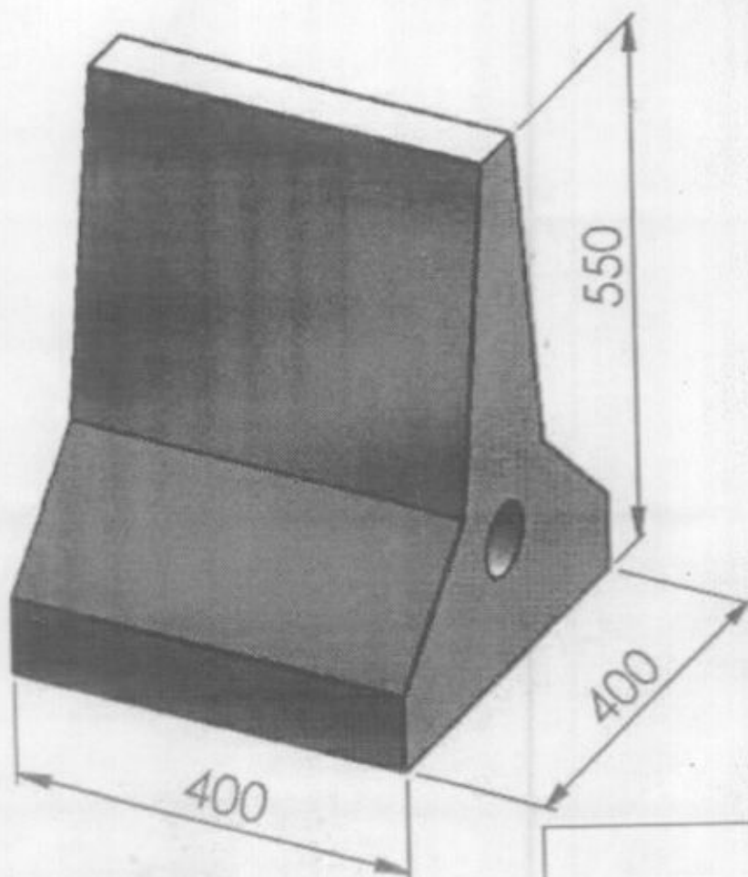
نیوجرسی بتنی شهری: ارتفاع ۵۵ اتصال با لوله
