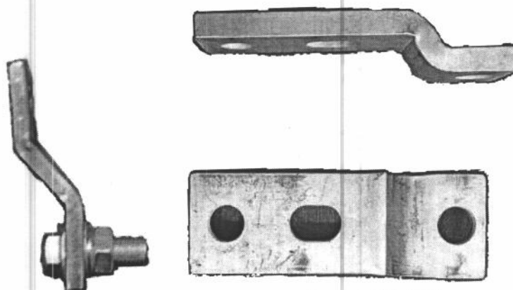
شکل (۲): نمونه‌هایی از شینه کمکی غیر هم‌سطح
