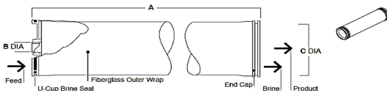
شکل شماره ۱. شماتیک مشخصات ممبران
