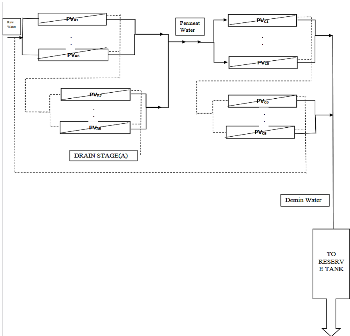
شکل شماره ۲. شماتیک تصفیه خانه RO
